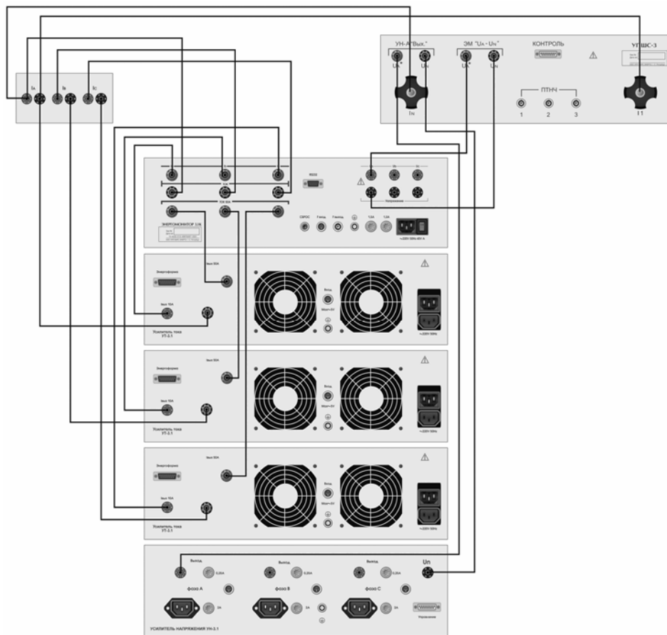
Рис. 1. Схема подключения УПШС-3 к установке «УППУ-МЭ 3.1КМ-С»
