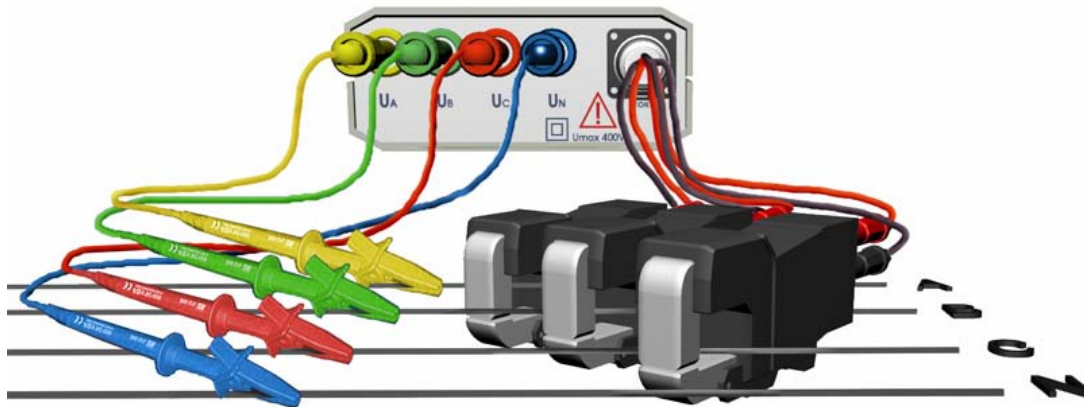
Рис. А.1. Схема подключения Прибора ПЭМ-02 к трехфазной четырехпроводной сети
