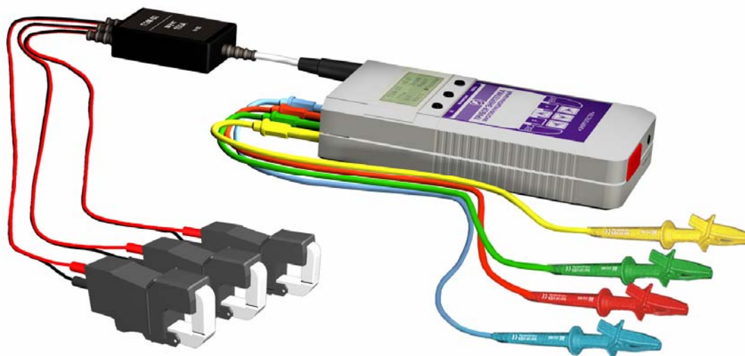
Рис. А.4. Схема подключения токоизмерительных клещей 10 (100) А к Прибору ПЭМ-02 через шунт I_H = 10 А для клещей 10 А (шунт I_H = 10 или 100 А для клещей 100 А)
