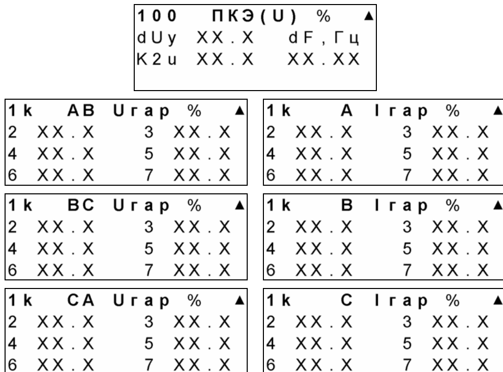
Рис. 4.11. Экраны режима отображения ПКЭ для трехфазной трехпроводной схемы подключения
