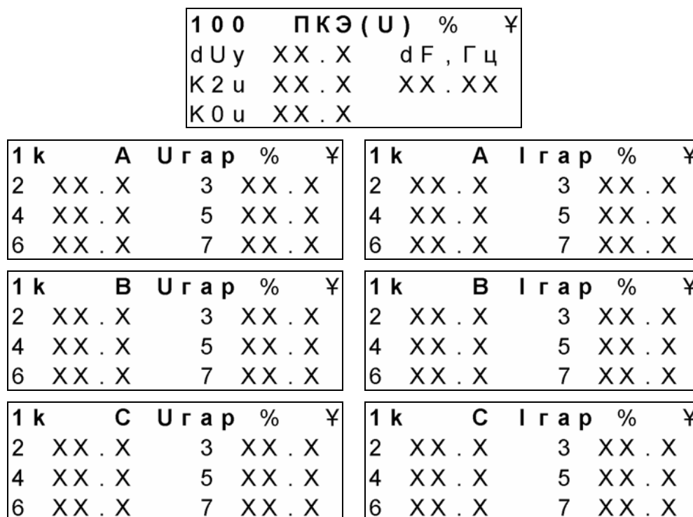
Рис. 4.10. Экраны режима отображения ПКЭ для трехфазной четырехпроводной схемы подключения
