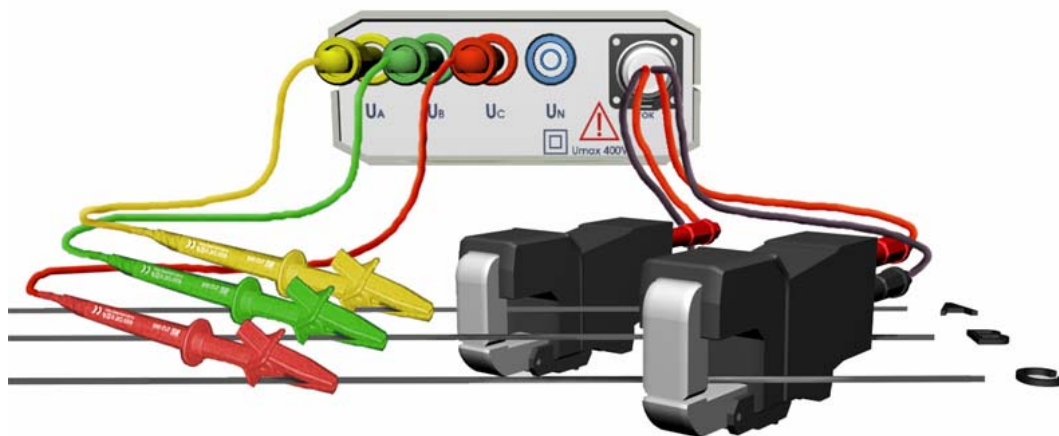
Рис. А.2. Схема подключения Прибора ПЭМ-02 к трехфазной трехпроводной сети
