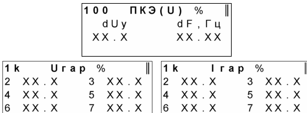
Рис. 4.12. Экраны режима отображения ПКЭ для однофазной двухпроводной схемы подключения
