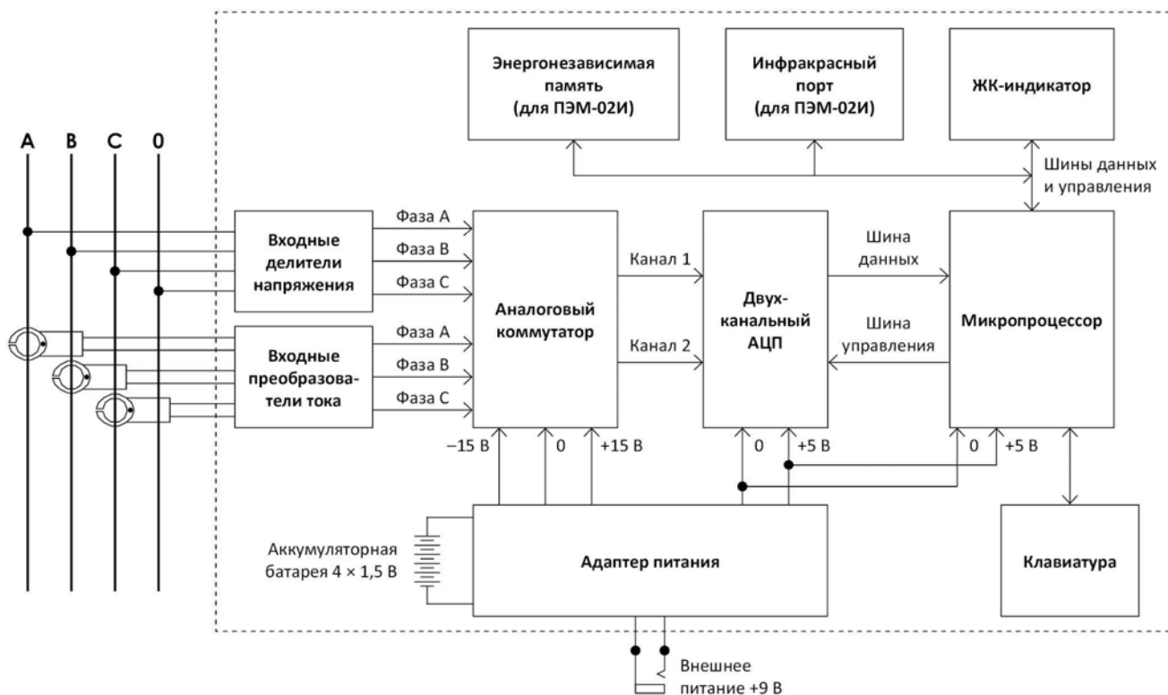
Рис. 2.1. Структурная схема Прибора ПЭМ-02
