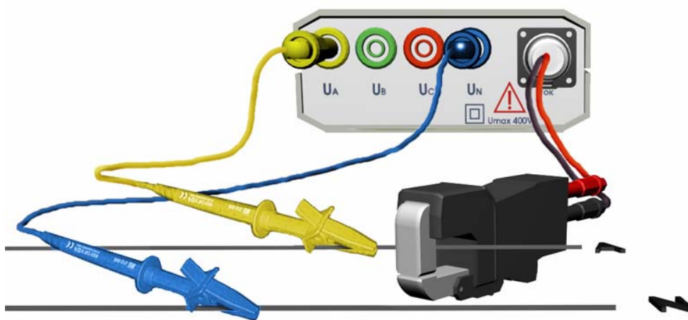
Рис. А.3. Схема подключения Прибора ПЭМ-02 к однофазной двухпроводной сети
