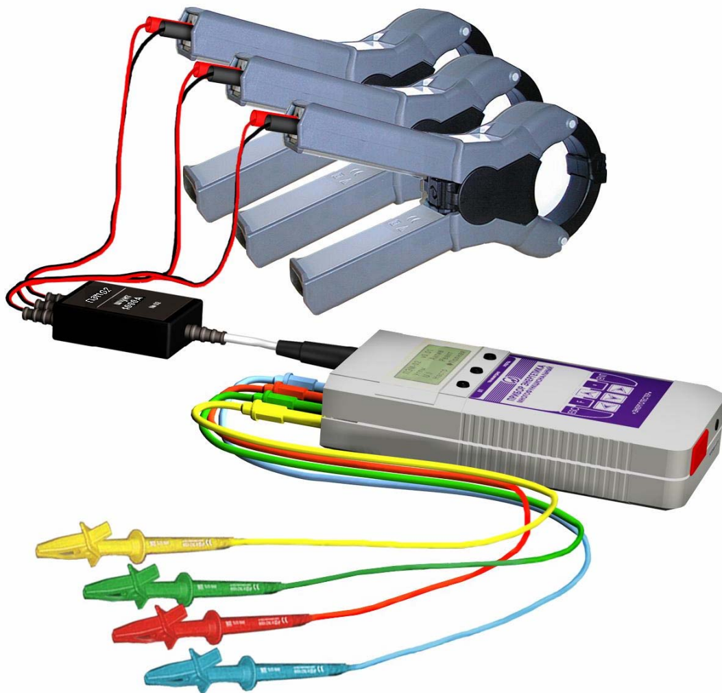
Рис. А.5. Схема подключения токоизмерительных клещей 1000 А к Прибору ПЭМ-02 через шунт I_n = 100 (1000) А для клещей 1000 А
