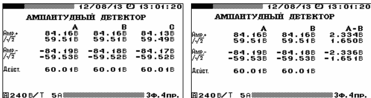
Рис. 4.55. Отображение разностных амплитудных значений напряжения в режиме «АМПЛИТУДНЫЙ ДЕТЕКТОР»
