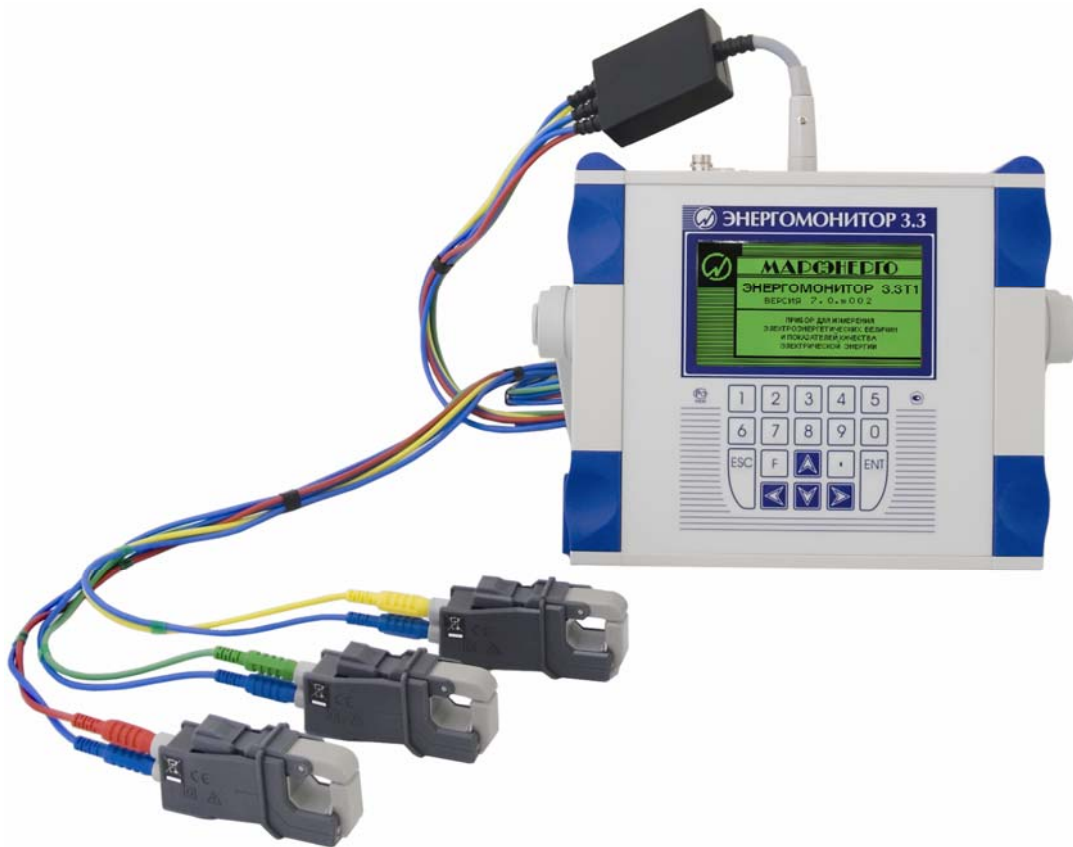
Рис. Б.1. Схемы подключения токоизмерительных клещей 10 А и 100 А к Прибору ЭМ-3.3Т1 с помощью Кабеля измерительного «Ток-К»
