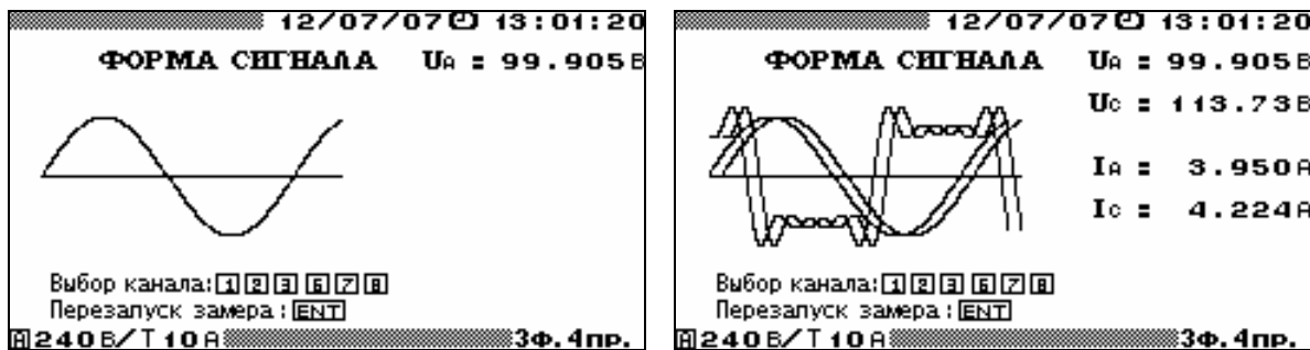
Рис. 4.13. Режим отображения формы сигнала
