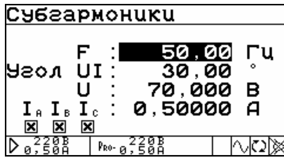
Рис. 4.16. Окно задания параметров субгармоник
