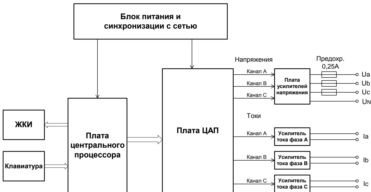
Рис. 2.2. Структурная схема Источника
